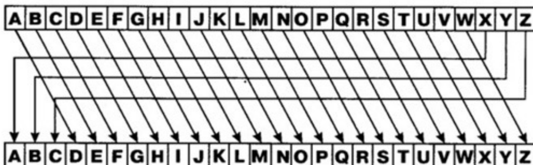
Рис. 2.3. Шифр Цезаря
